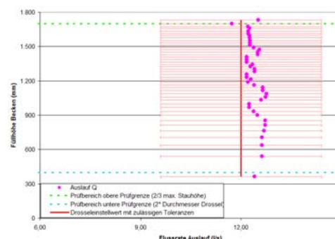
Qh- Plot der Parameter Füllhöhe Becken und Flussrate im Auslauf
